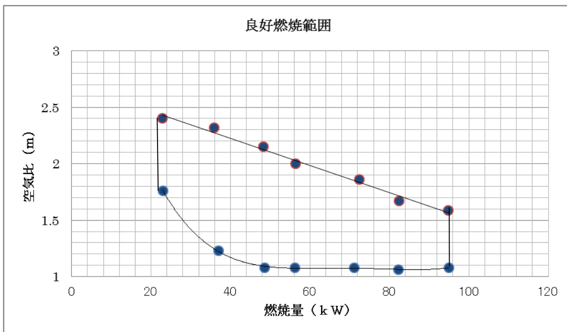
熱交付（最低燃焼予熱空気温度約150℃ 最大燃焼予熱空気温度約230℃のデータ）
