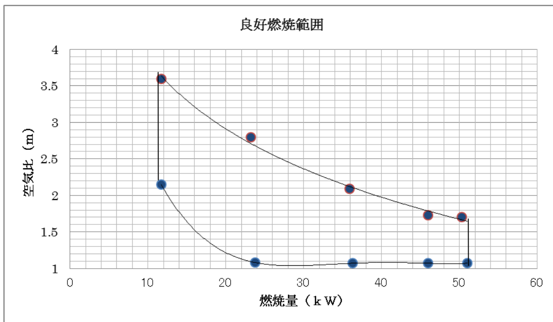
熱交付 (最低燃焼予熱空気温度約150°C 最大燃焼予熱空気温度約230°Cのデータ)
