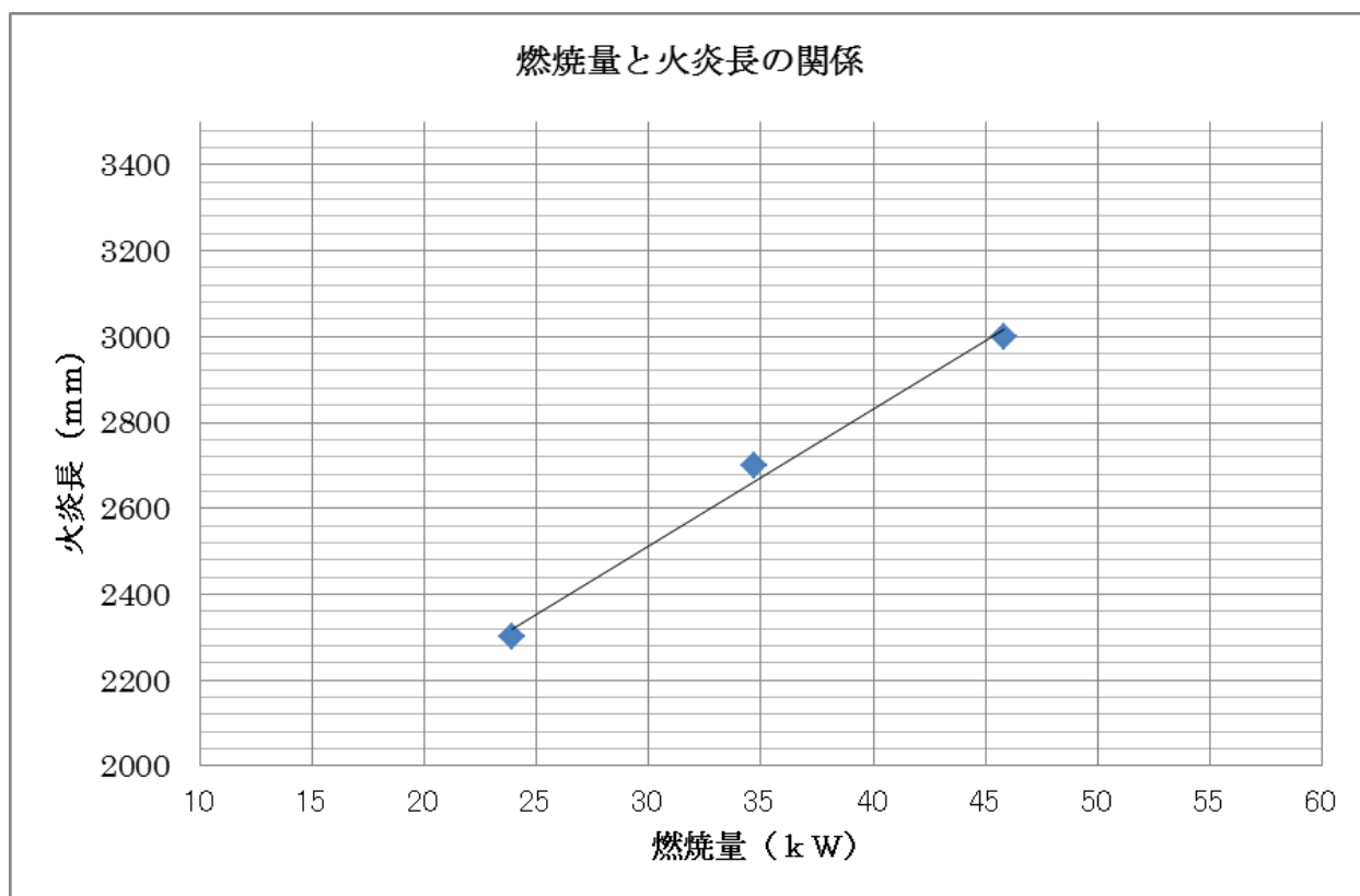
空気比 = 1.1 熱交なし
