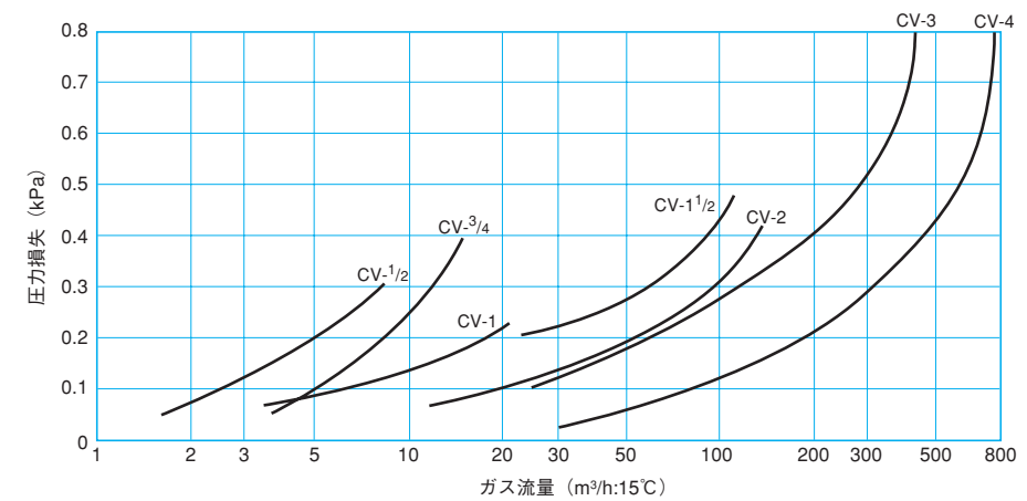
(データ) ガス流量 (13A比重0.65) と圧力損失の関係 (水平取付)
